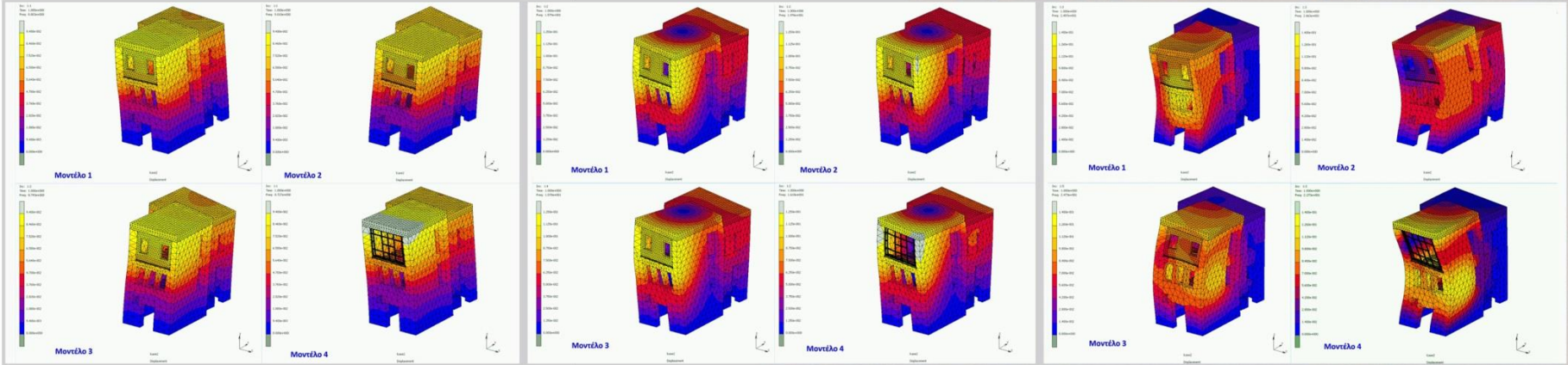
Δυναμική ιδιομορφική ανάλυση των μοντέλων σε τρεις ιδιοσυχνότητες - Dynamic modal analysis of examined models ( Displacements at three eigenfrequencies)
